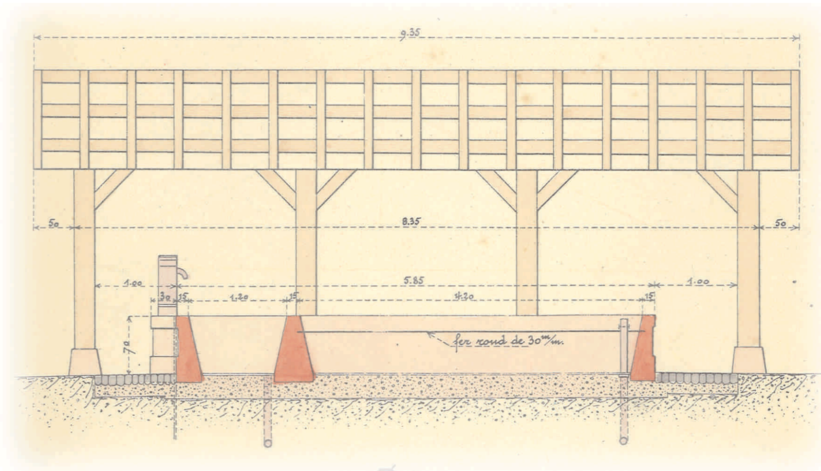
Détail du plan de coupe longitudinale - projet de 1922
